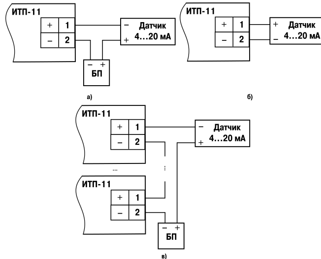
Рисунок 8.1 - Схемы подключения: а) подключение ИТП-11 к пассивному источнику 4...20 мА; б) подключение ИТП-11 к активному источнику 4...20 мА; в) подключение нескольких ИТП-11 к пассивному источнику 4...20 мА
